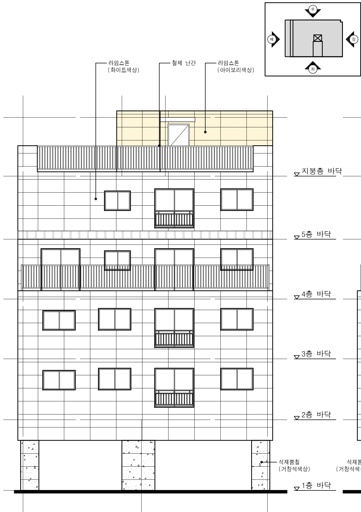
배면도 SCALE : A3 : 1/100
