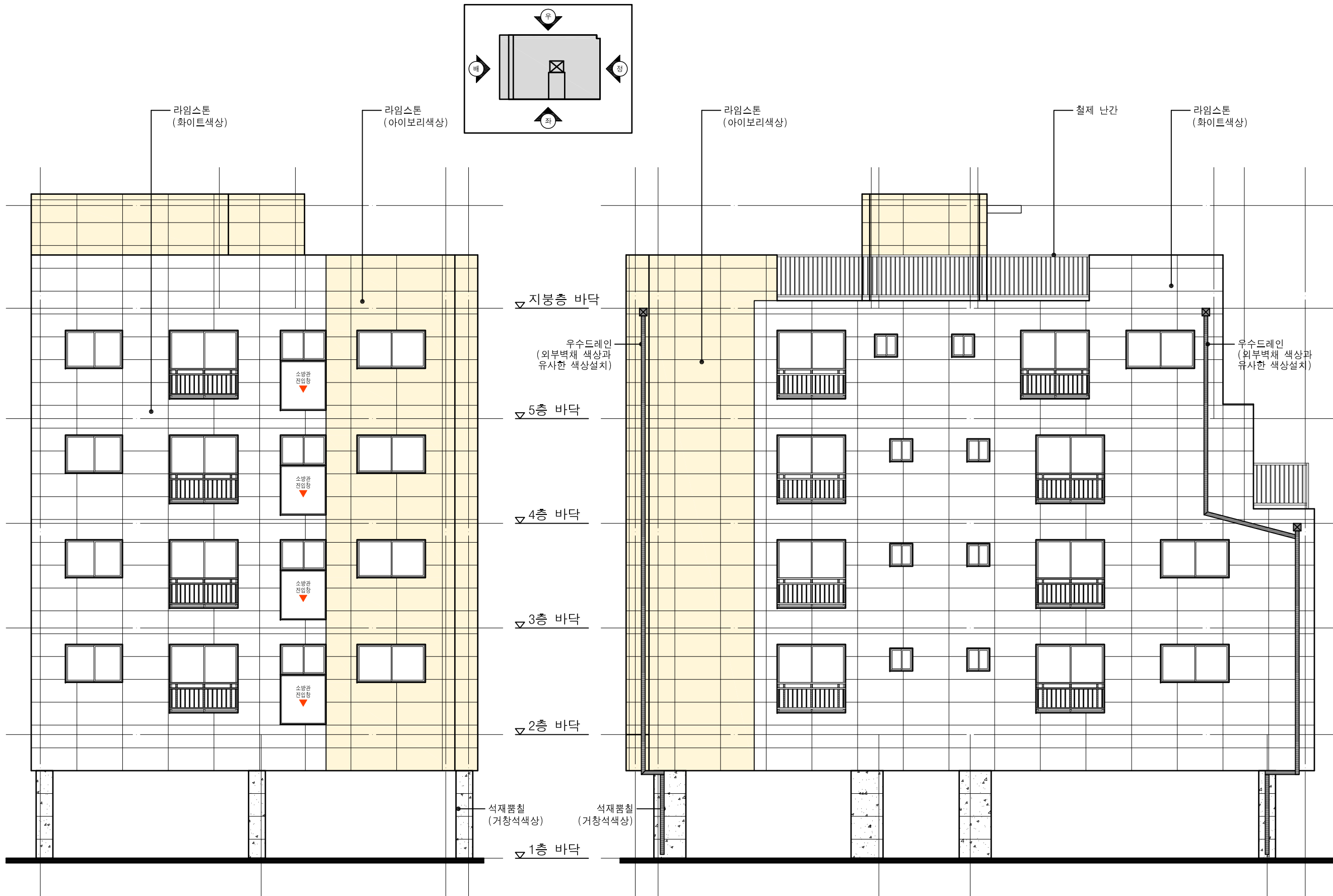
정면도 SCALE : A3 : 1/100
