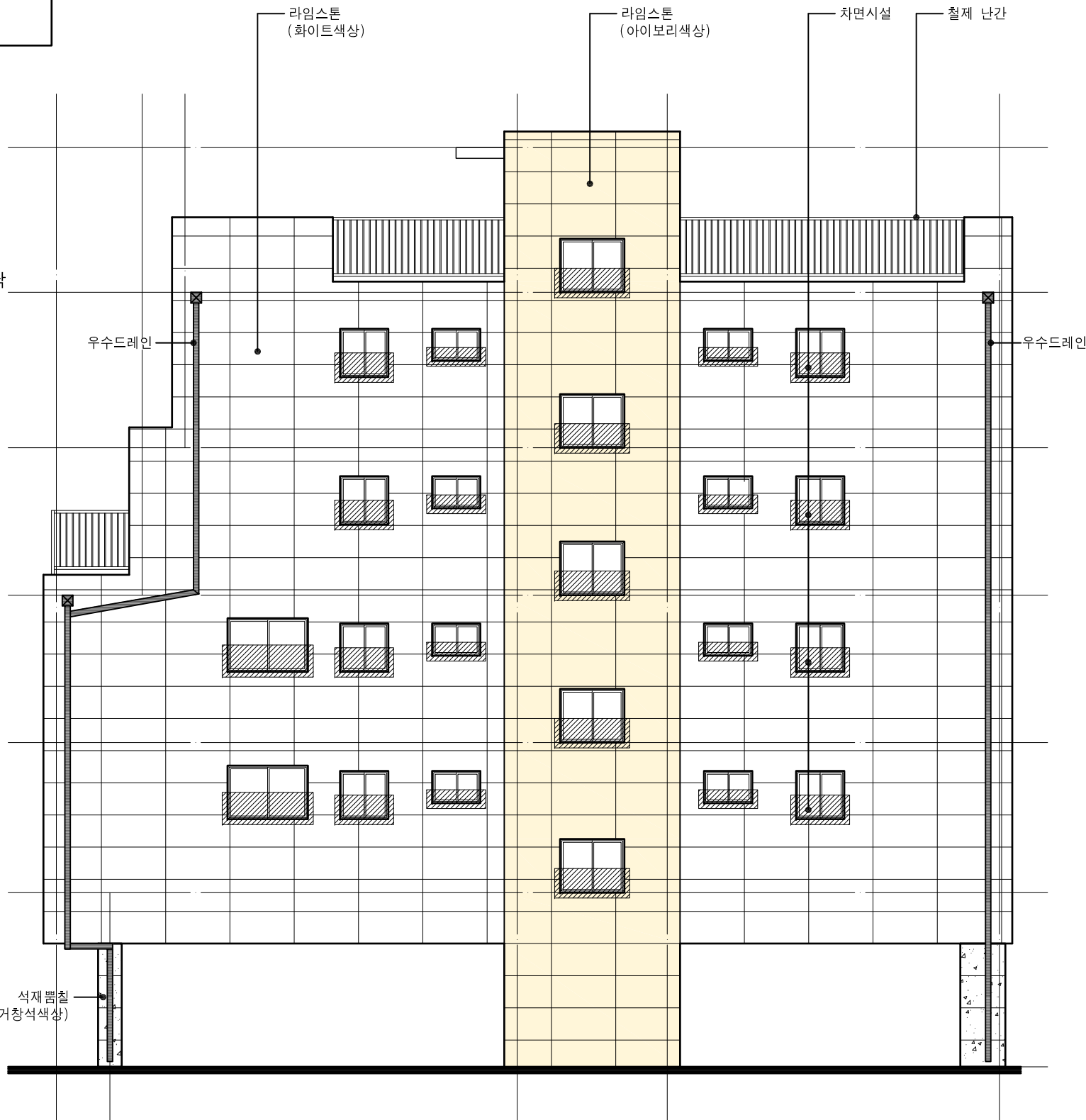
좌측면도 SCALE : A3 : 1/100
