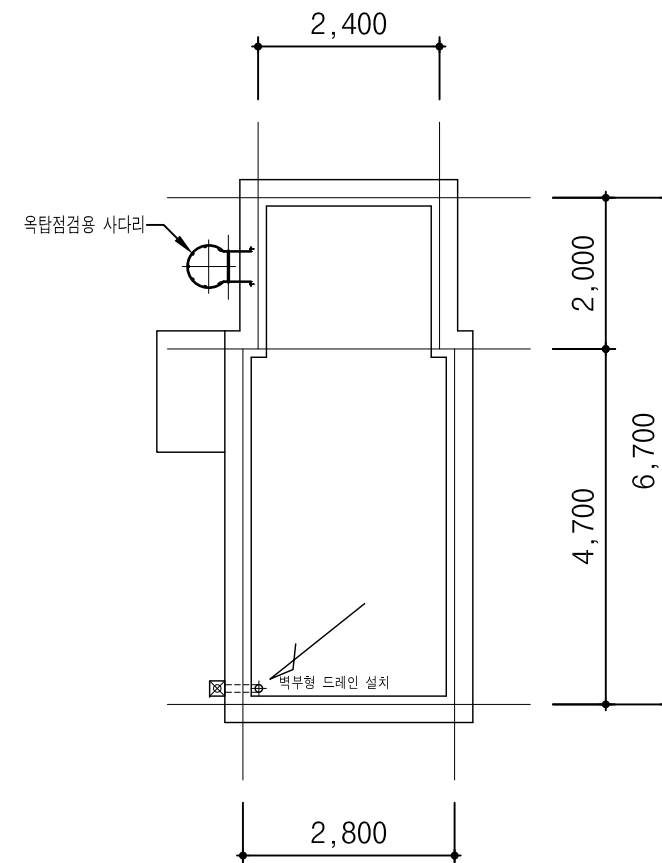
지붕및옥탑평면도 SCALE : A3 : 1/100
